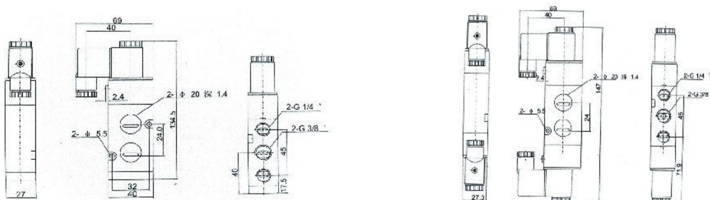
外观尺寸 (图 )
